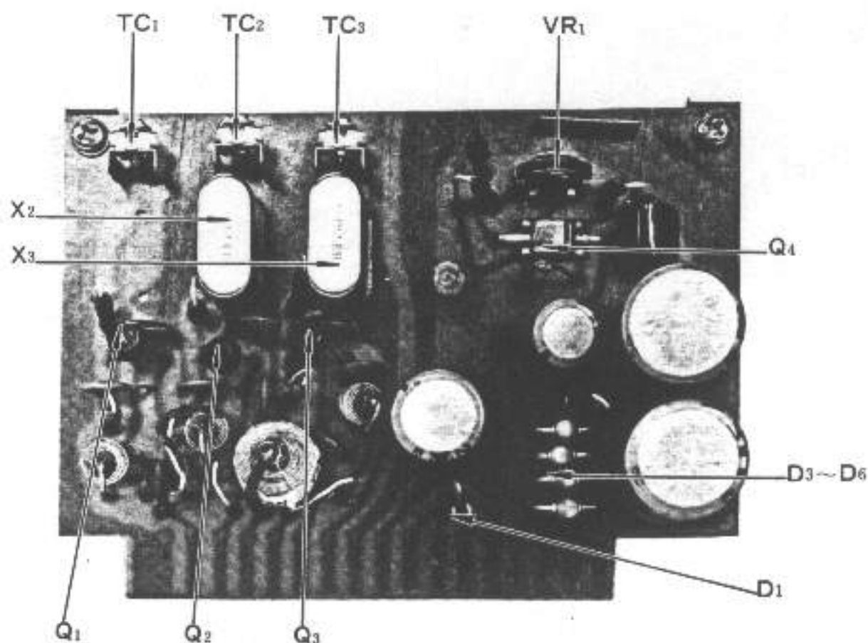
Fig. 17 REG-BFO UNIT
