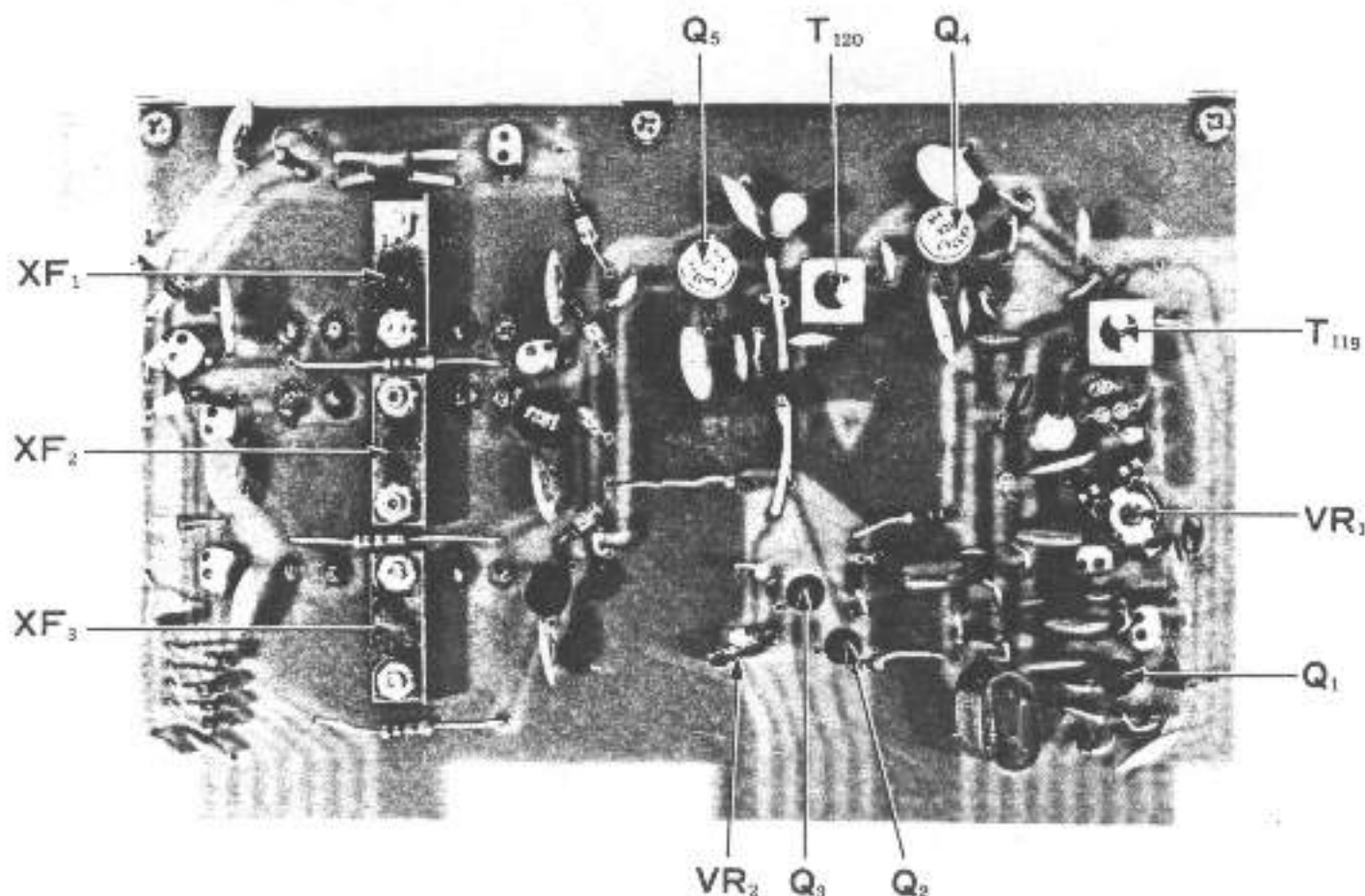
Fig. 15 IF UNIT
