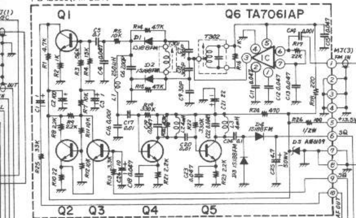
PB-1269C(FM DET)
